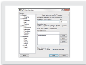
[ PuTTY ]
